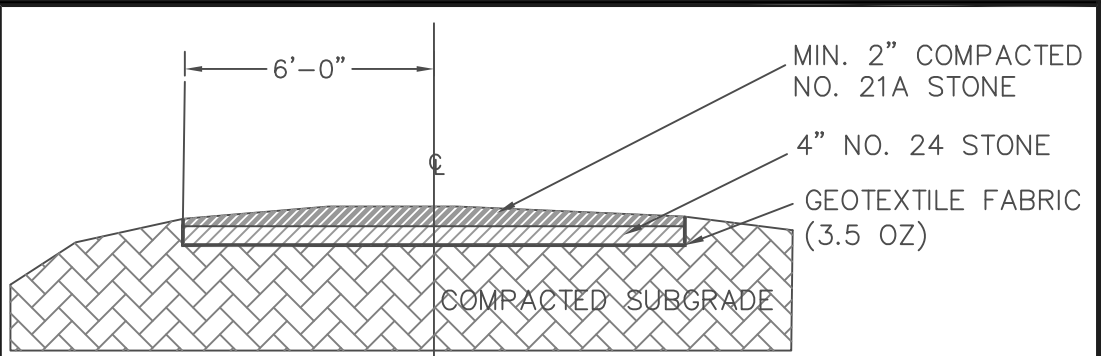
ACCESS ROAD SECTION N.T.S.
